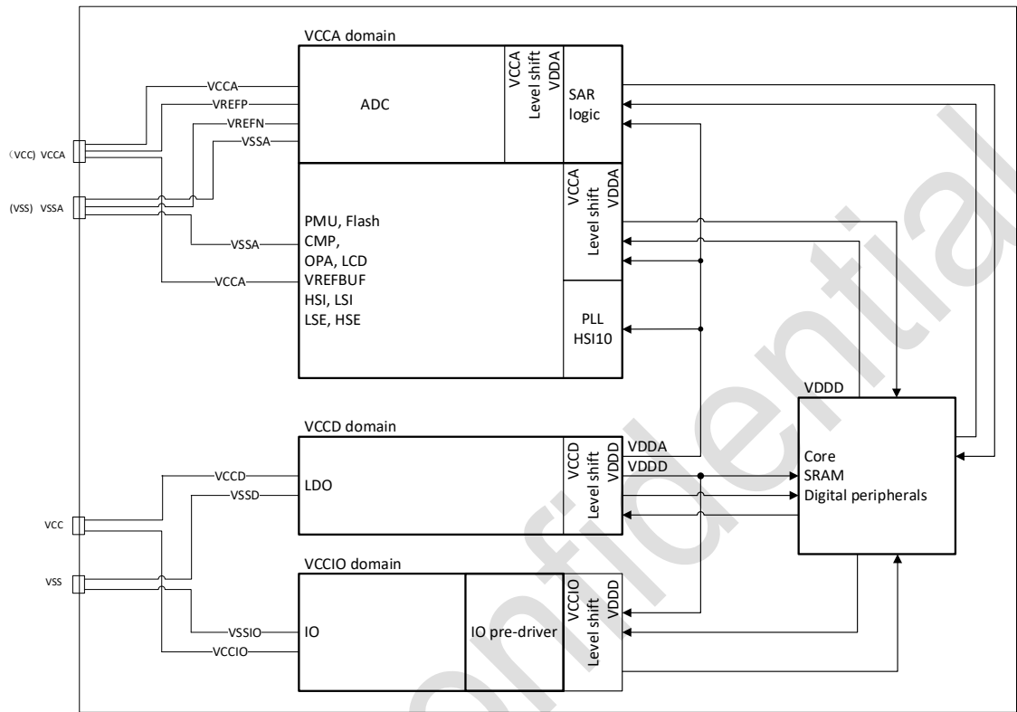
图 2-2 电源框图
