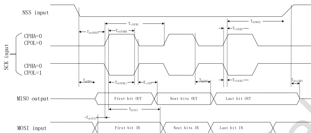
图 5-3 SPI 时序图-slave mode 和 CPHA=0
