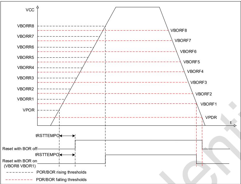
图 2-3 POR/PDR/BOR 阈值
